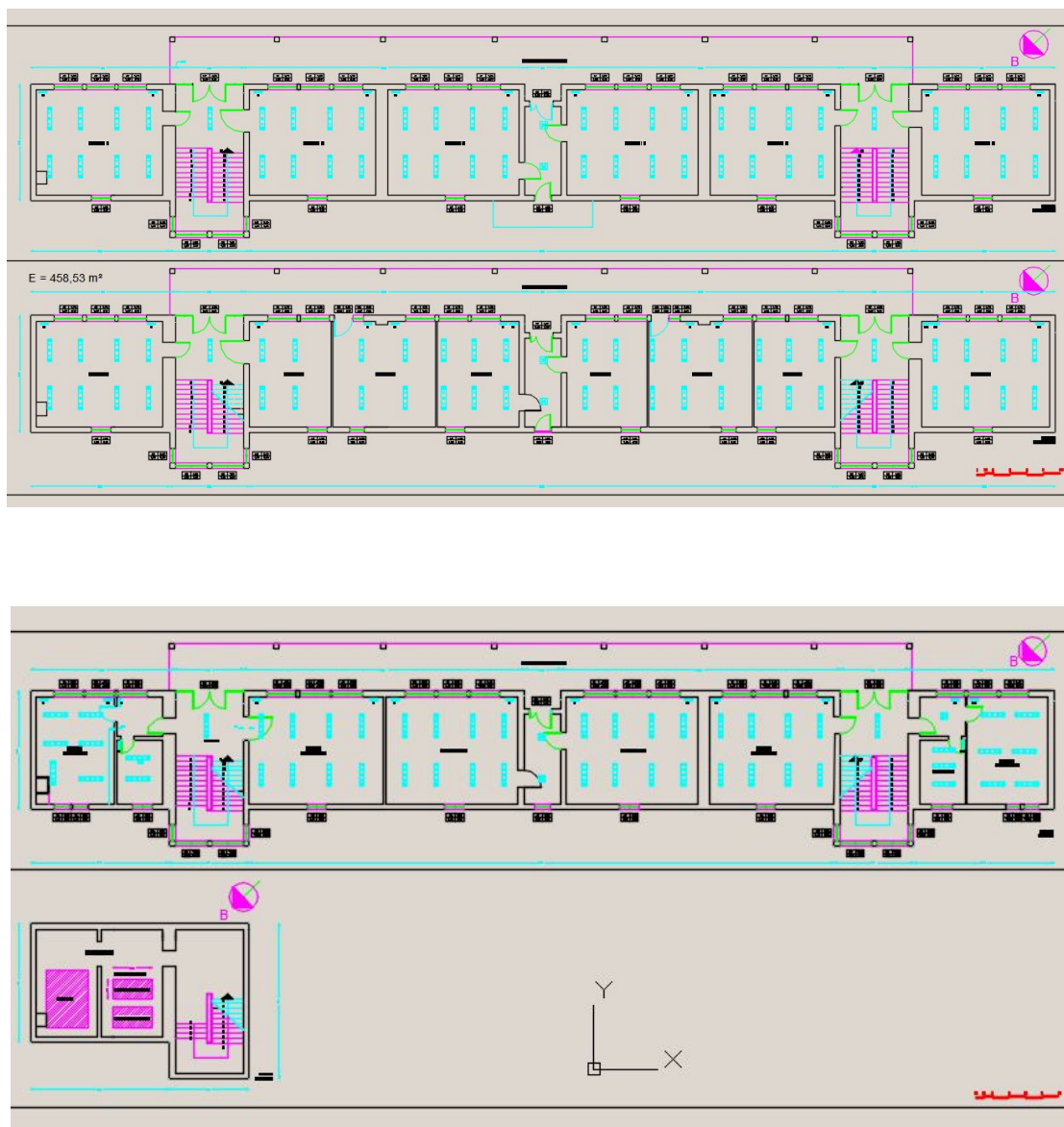
Σχήμα 4.1β: Κατόψεις κτιρίου
