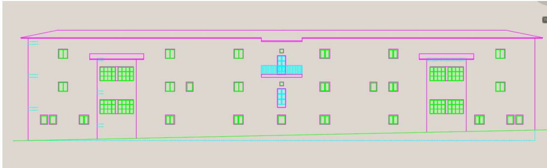
Σχήμα 4.1α: Όψεις κτιρίου
