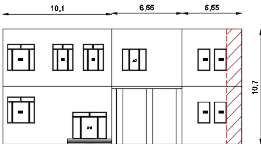
Σκαρίφημα Ανατολικής Όψης
