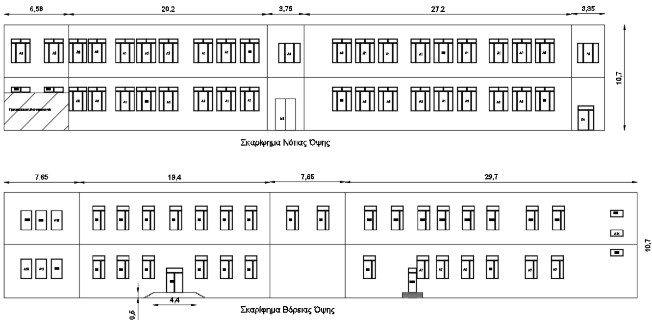
Σχήμα 4.1α: Όψεις κτιρίου
