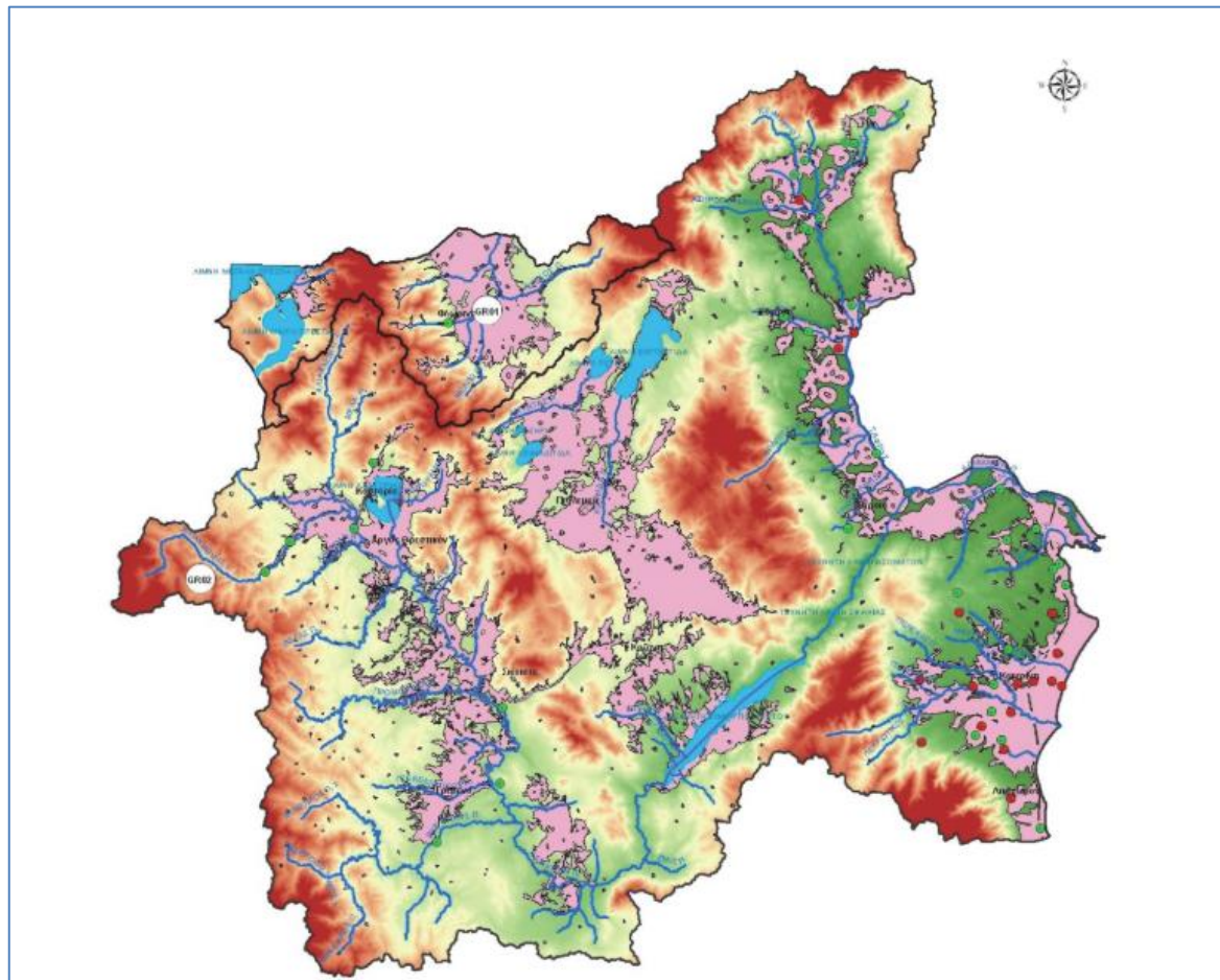
Χάρτης 5: Ζώνες Δυσνητικά Υψηλού Κινδύνου Πλημμύρας ΥΔ 09
