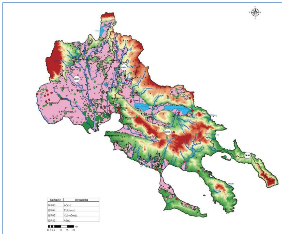
Χάρτης 6: Ζώνες Δυσνητικά Υψηλού Κινδύνου Πλημμύρας ΥΔ 10
