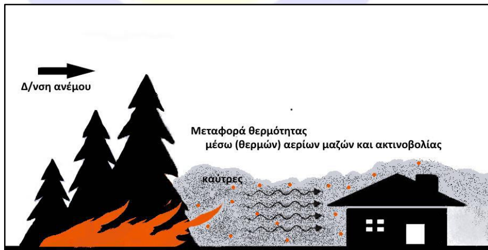
Σχέδιο 4. Τρόποι ροής της θερμότητας σε μια δασική πυρκαγιά, που εξελίσσεται πλησίον κτιρίου και απεικόνιση πιθανού τρόπου
